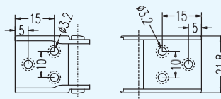
10×15接头
