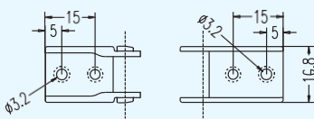
10×20接头
