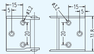
10×25接头
